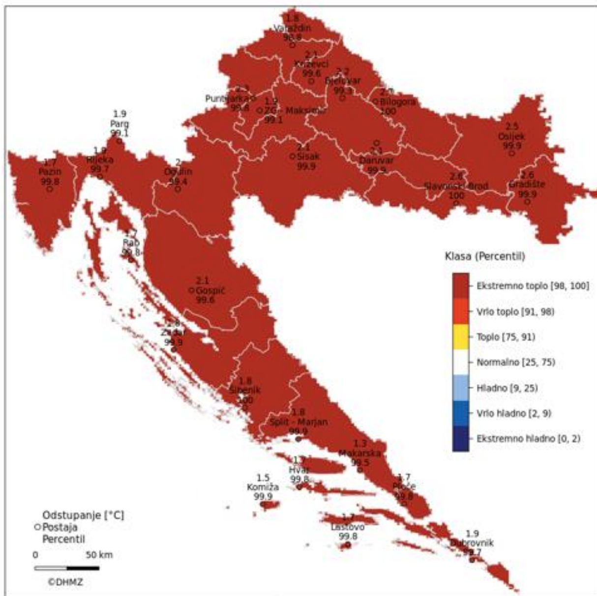
Godina 2024. Srednja temperatura zraka Percentili u odnosu na normalu 1991.-2020.
