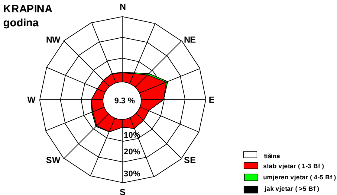
Slika 4: Godišnja i sezonske ruže vjetra, Krapina, 1993–2000.
