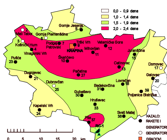
Slika 5: Prostorna raspodjela srednjeg broja dana s tučom i/ili sugradicom za vrijeme sezone obrane od tuče. Krapinsko-zagorska županija, 1981.–2000.
